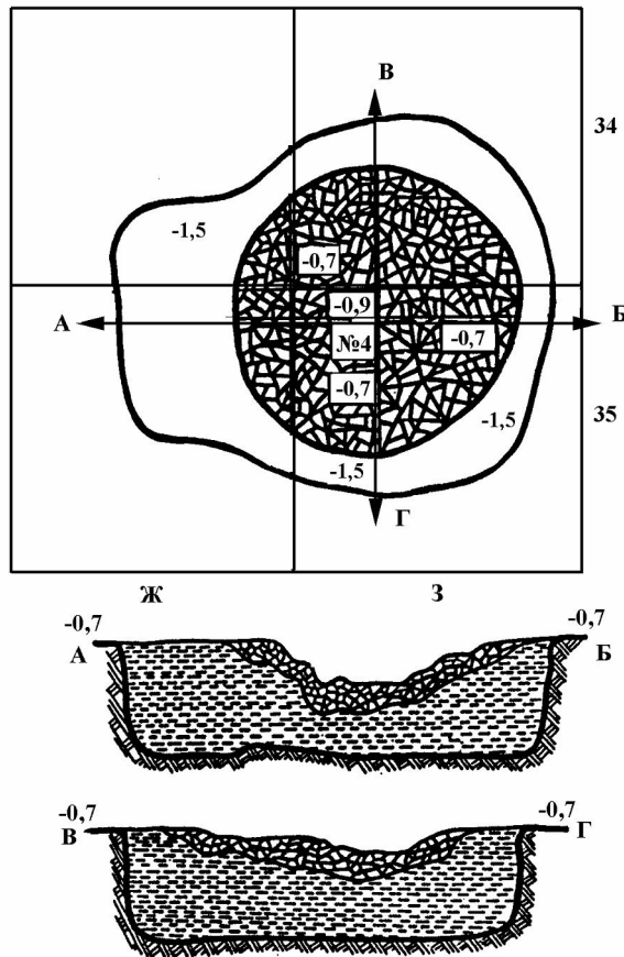
Рис. 4. Тарасівка. 1978. Ур. Підліс. План та переріз ями № 4
