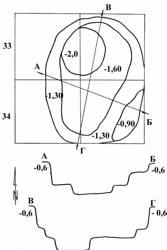
Рис. 3. Тарасівка. 1978. Ур. Підліс. План і перерізи житла III Fig. 3. Tarasivka. 1978. Place Pidlis. Plan and cross-sections of dwelling III
