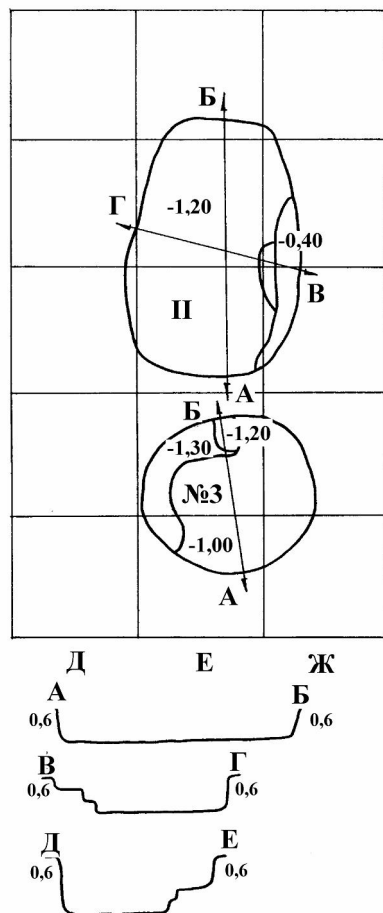
Рис. 2. Тарасівка. 1978. План і перерізи житла II та ями № 6 Fig. 2. Tarasivka. 1978. Plan and cross-sections of dwelling II and pit № 6
