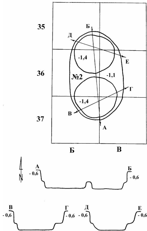
Рис. 5. Тарасівка. 1978. Ур. Підліс. План та перерізи ями № 2 Fig. 5. Tarasivka. 1978. Place Pidlis. Plan and cross-sections of pit № 2
