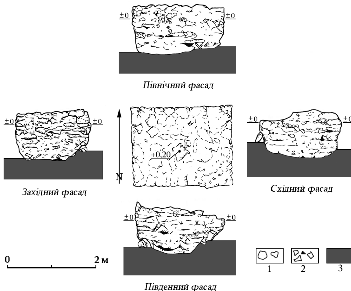
Рис. 7. Звенигород. Окольный город. Східна частина. План і фасади кам'яного стовпа (рис. за О. Ратичом). Умовні позначення: 1 – камінь, 2 – подрібнена цегла, 3 – материк
