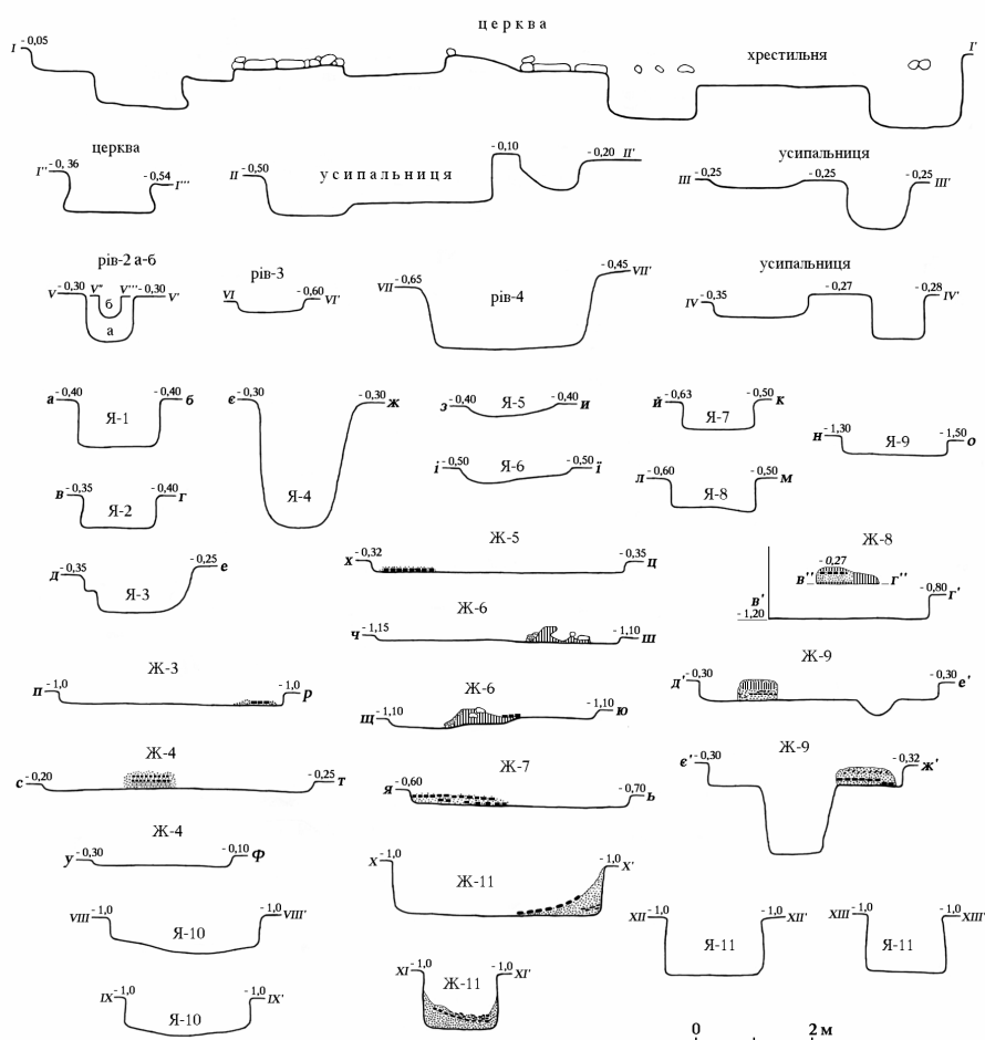
Рис. 4. Звенигород. Окольный город. Східна частина. Переріз об'єктів у секторі IV (рис. за О. Ратичом)
