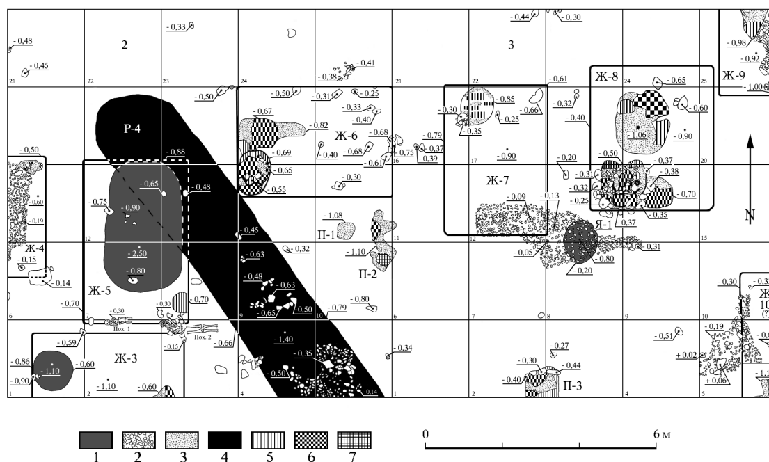
Рис. 8. Звенигород. Окольний город. Східна частина. План розкопів у секторі II. Локалізація об'єктів (рис. за О. Ратичом). Умовні позначення: 1 – яма, 2 – каміння, 3 – печина, 4 – рів, 5 – глина, 6 – черинь, 7 – попіл. Об'єкти: Я – яма, Ж – житло, П – піч, Р – рів
