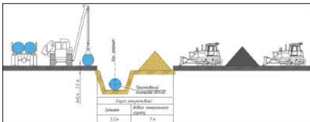
Рис. 2. Схема будівельної смуги магістрального газопроводу
