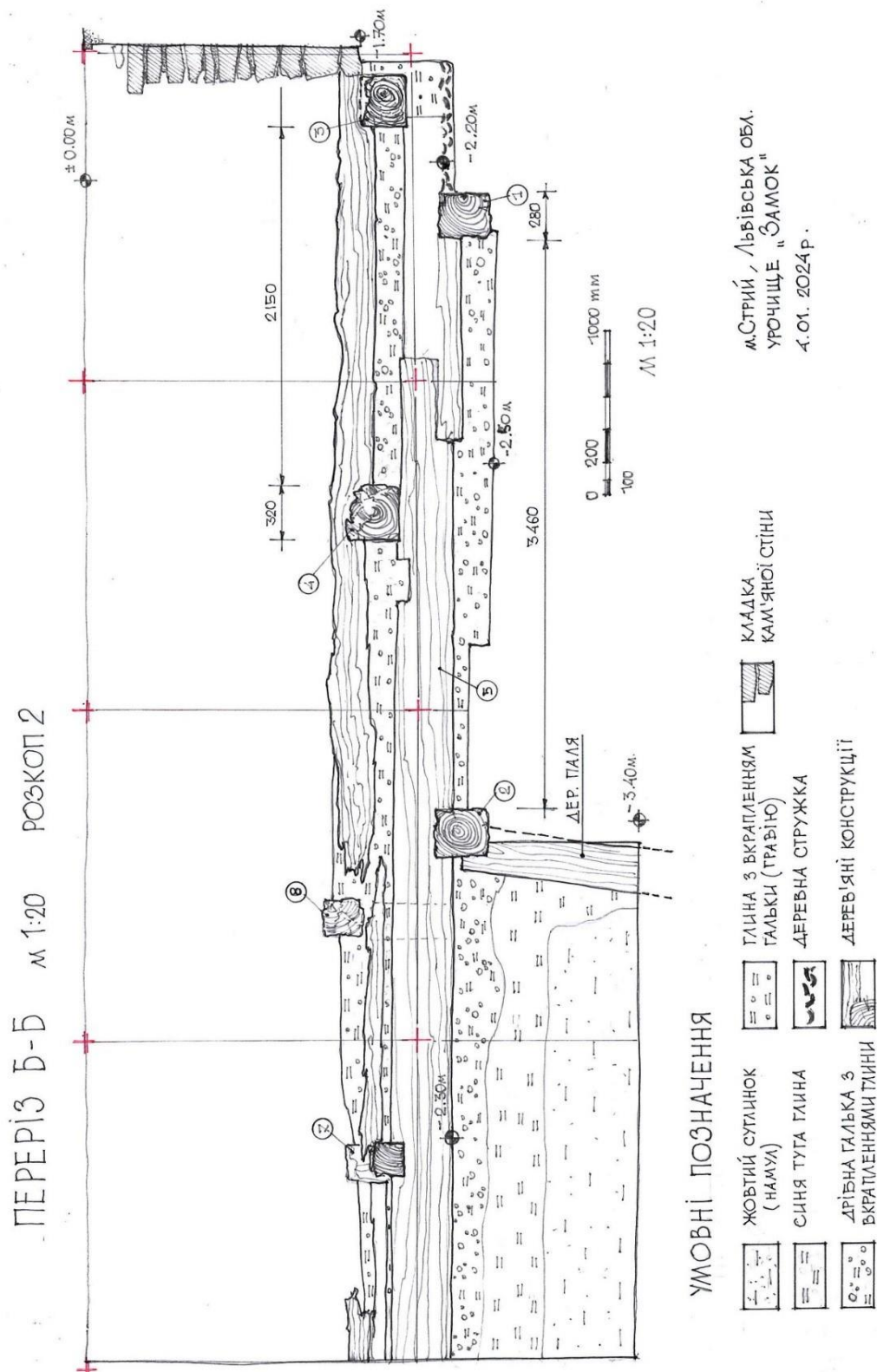
Рис. 5. Стрий, стратиграфічний переріз вздовж поздовжньої осі споруди-3 на розкопі-II Fig. 5. Stryi, stratigraphic section along the longitudinal axis of structure-3 in excavation-II
