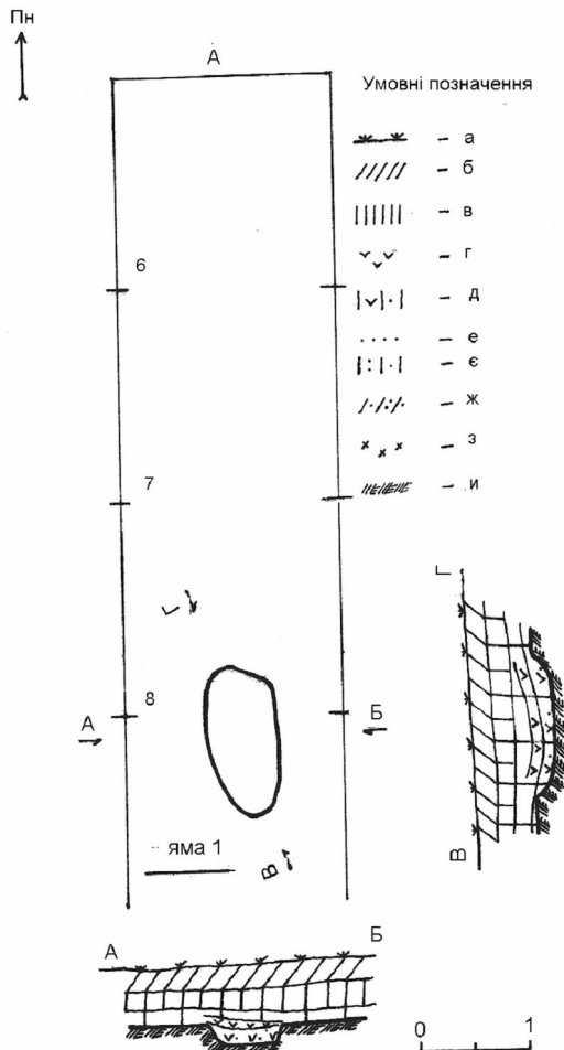
Рис. 4. Яма 1. Умовні позначення: а – сучасна поверхня, б – сірий гумус, в – темно-сірий перехідний шар, г – вугілля, д – чорний вуглистый шар, е – пісок, є – сіро-коричневий шар (органіка, лімоніт), ж – темний коричнево-білесий шар (лімоніт, вапняк), з – глина (каолін), и – материк (супісок)
