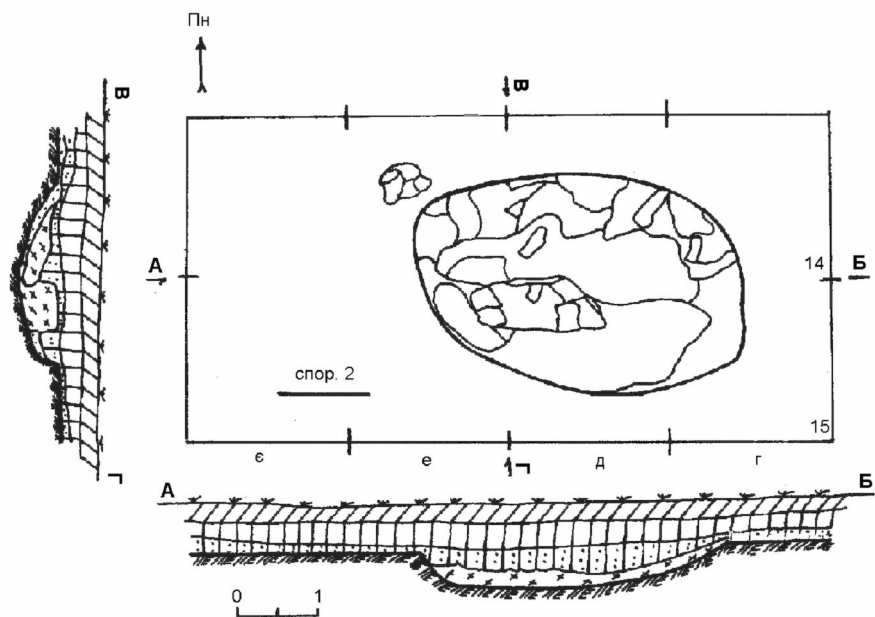
Рис. 8. Споруда 2 Fig. 8. Building 2
