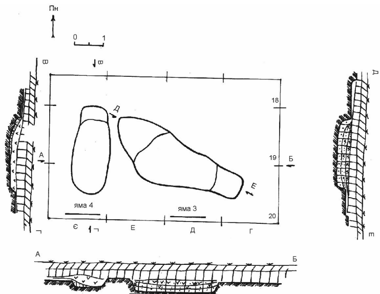
Рис. 6. Ями 3 і 4 Fig. 6. Pits 3 and 4
