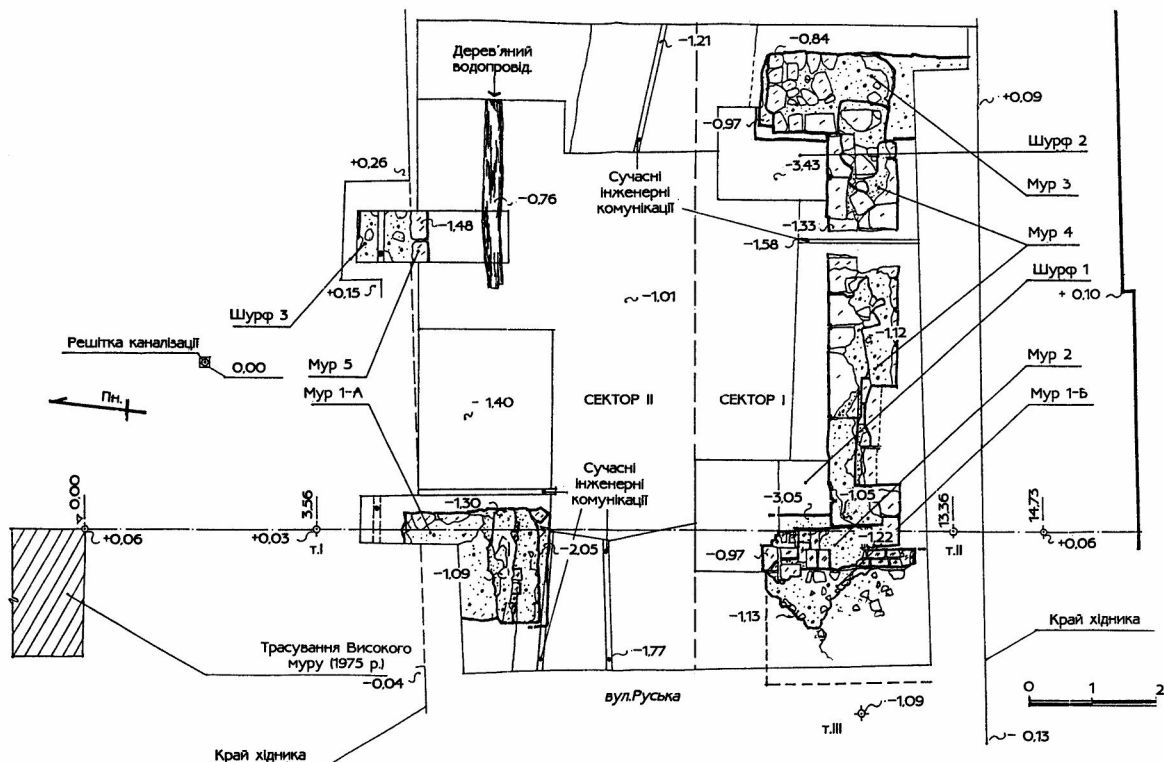
Рис. 2. План розкопу на Руській Fig. 2. Plan of the excavated area in Rus'ka street
