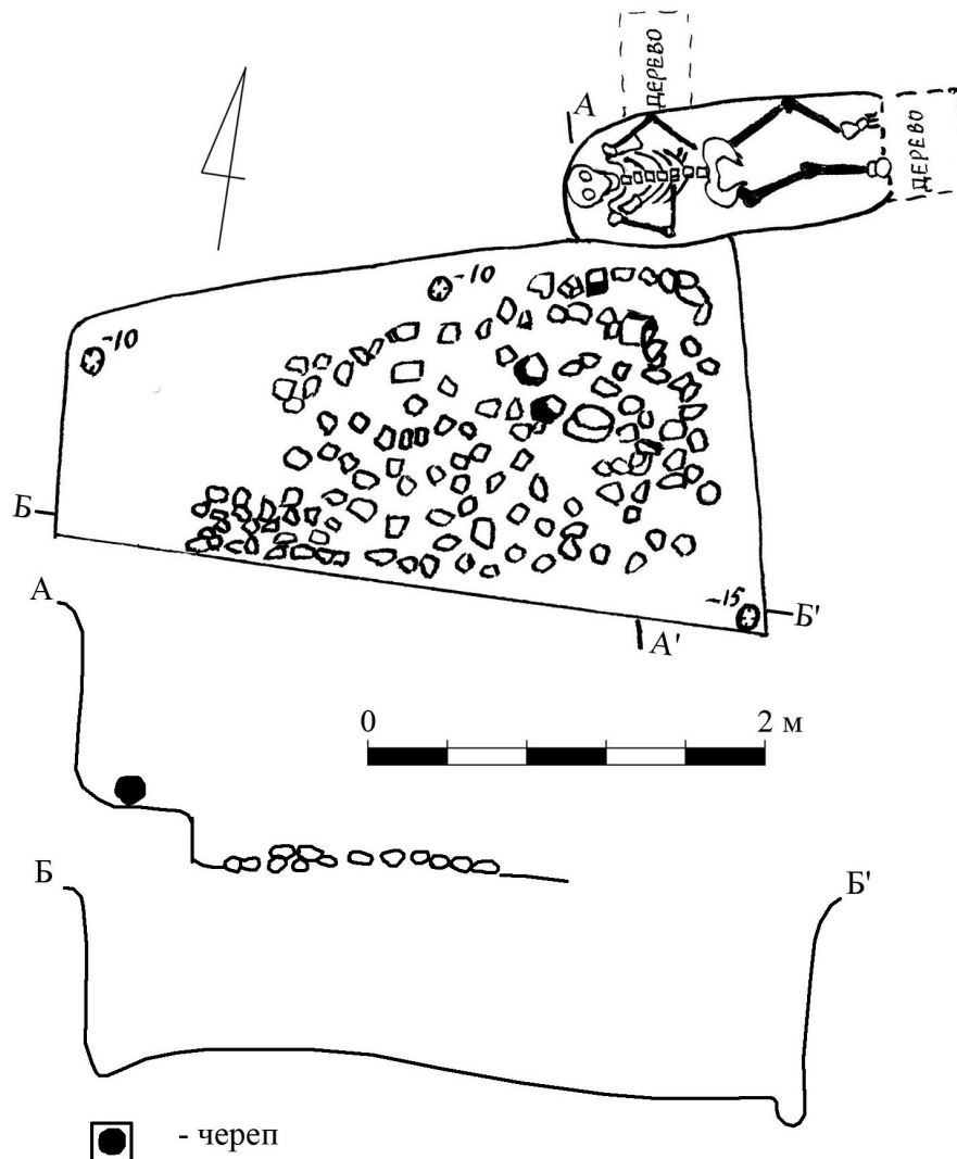
Рис. 5. План та профіль культової споруди X ст. (за: М. Ягодинська, 1987)
