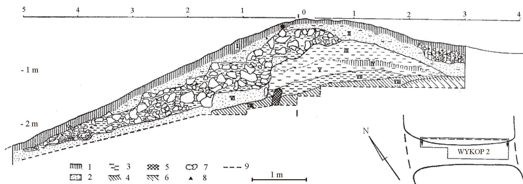
Rys. 3. Guciów, stan. 7. Ceramika i przekrój (sciana NE) wału grodziska. Badania 1971 – 1972 (wg. H. Zoll-Adamikowej, 1974). 1 – humus współczesny; 2 – piasek; 3 – glina; 4 – siwoszara glina; 5 – próchnica (śląd słupa?); 6 – piaszczysty calec; 7 – kamienie wapienne; 8 – miejsce znalezienia brzegu naczynia; 9 – poziom dna wykopy
