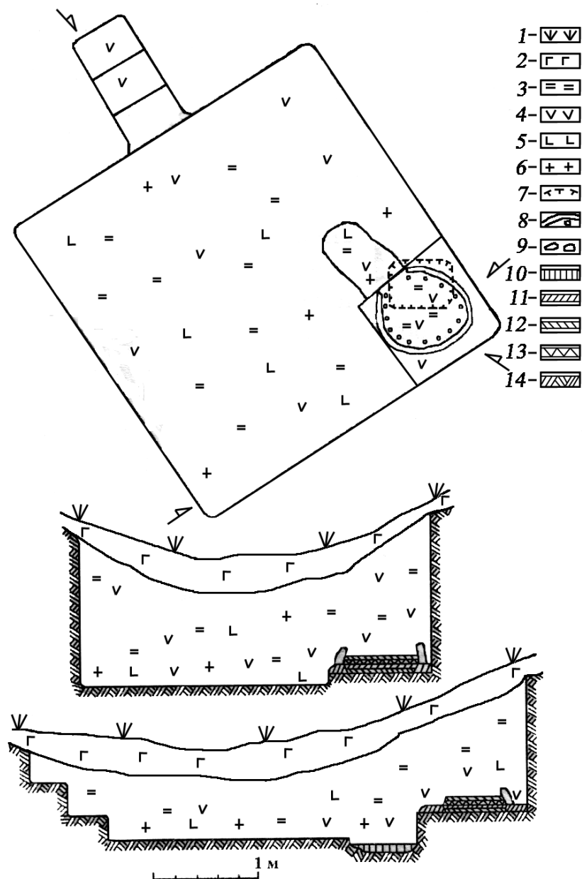
Рис. 2. План та перерізи напівземлянки XII – першої половини XIII ст. з Чорнівського городища. 1 – трава; 2 – гумус; 3 – обпалена земля; 4 – вугілля; 5 – кераміка; 6 – кістки; 7 – контури черіня; 8 – стінки глинобитної печі із стовповими ямками; 9 – печина; 10 – яма з золою; 11 – глиняна підмазка черіня; 12 – черінь глинобитної печі; 13 – черінь глинобитної печі 2; 14 – материк
