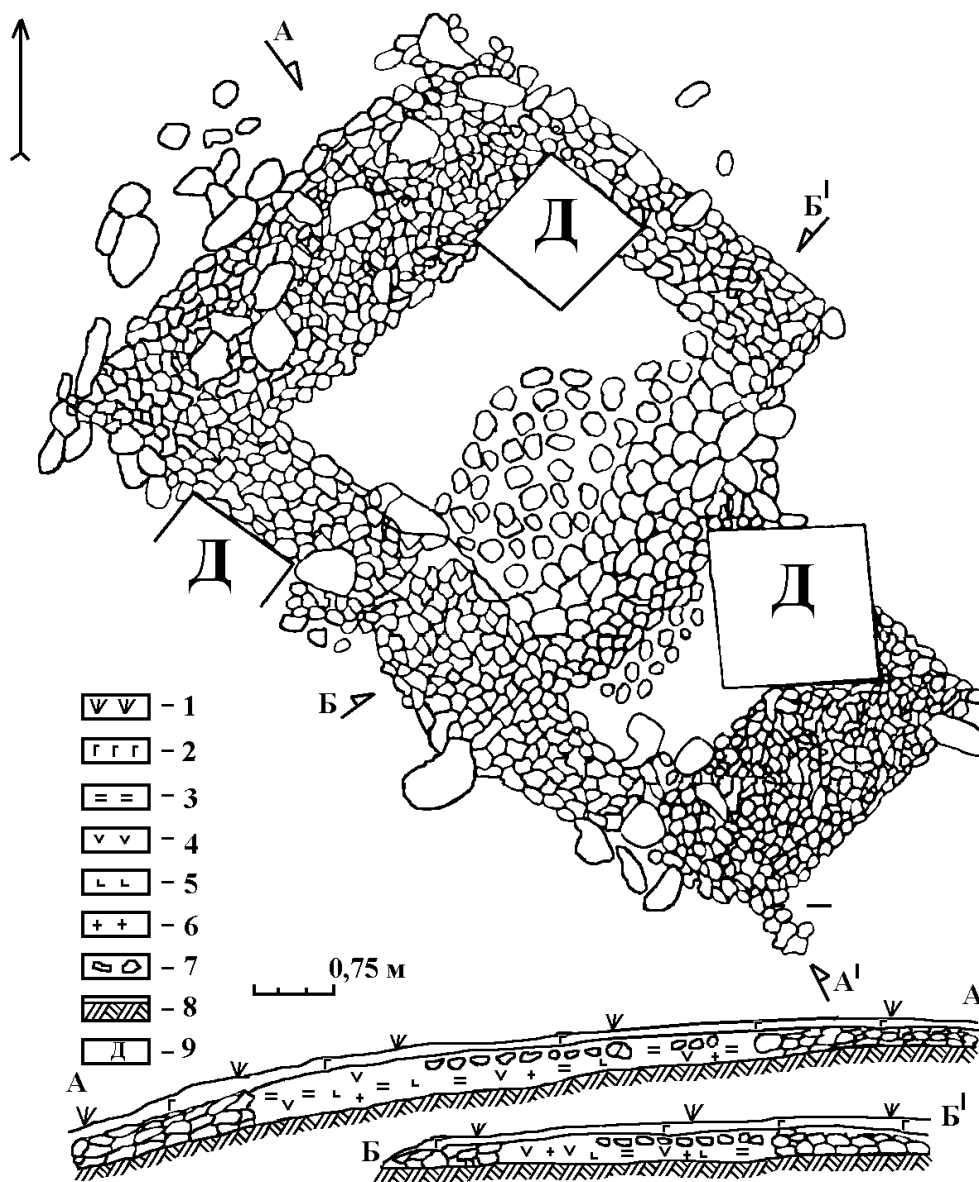
Рис. 8. План та профілі житла 4 з Чорнівського городища XII – першої половини XIII ст. 1 – трава; 2 – гумус; 3 – обпалена земля; 4 – вугілля; 5 – кераміка; 6 – кістки; 7 – каміння; 8 – материк; 9 – дерево Fig. 8. Plans and profiles of dwelling 4 from Chornivka hill-fort of XII – first half of XIII century. 1 – grass; 2 – soil; 3 – burned soil; 4 – coal; 5 – ceramics; 6 – bones; 7 – stones; 8 – mainland; 9 – tree
