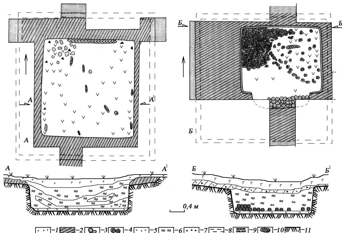
Рис. 7. Плани та профілі наземних жител з підвалами з городища X ст. Ревне 1 Б (за: Тимошук, 1982, с. 49, рис. 26). 1 – гумус; 2 – культурний шар – залишки будівлі; 3 – камені; 4 – обпалені камені; 5 – глина; 6 – вугілля; 7 – шматки обпаленої глини; 8 – реконструкція зрубів; 9 – ровик – відбиток нижньої колоди зрубу; 10 – обгоріле дерево; 11 – материк
