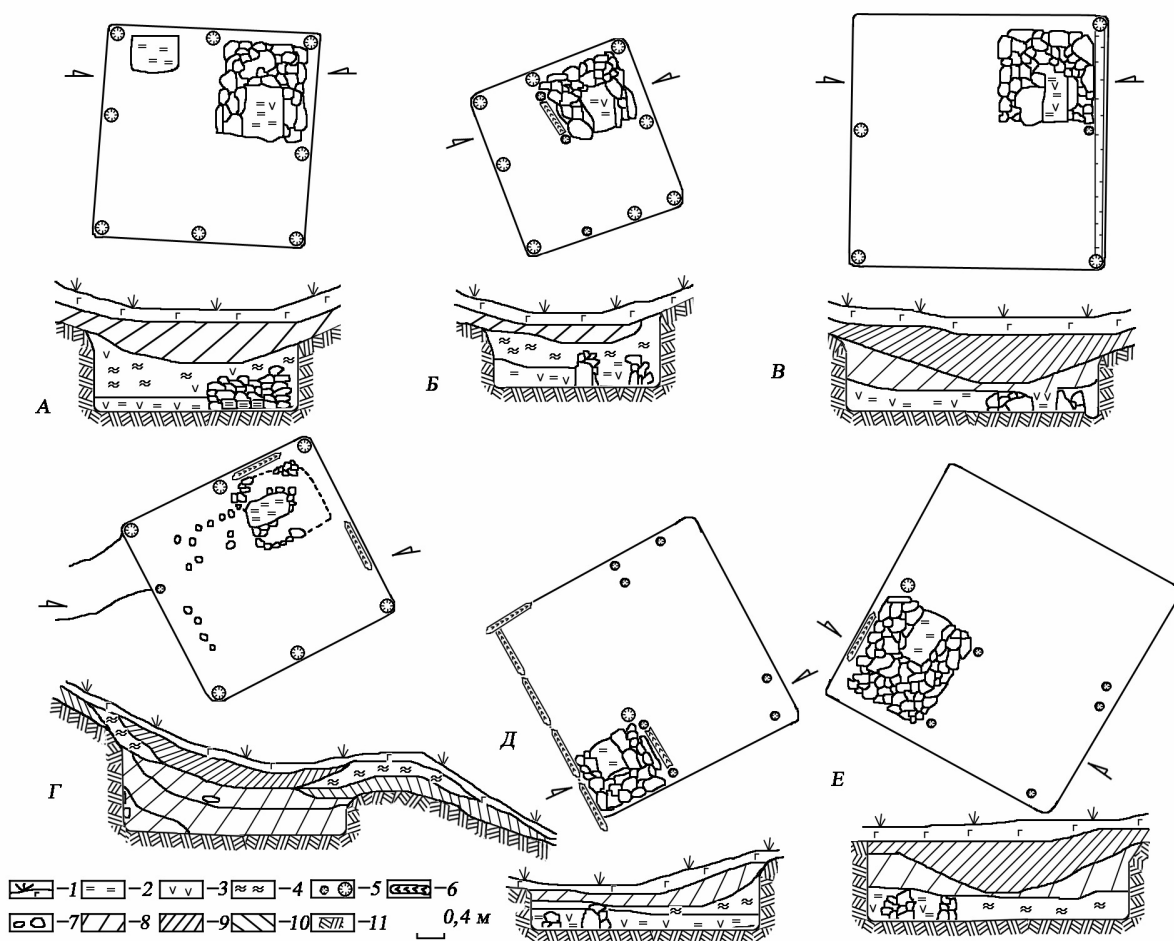
Рис. 1. Напівземлянкові житла X–XI ст. А – Г – житла зі стінами каркасно-стовпової конструкції; Д–Е – житла зі стінами зрубної конструкції. А – Ревне, житло №4; Б – Біла, житло №2; В – Цецин, житло №1; Г – Коростувата 3; Д – Коростувата 1, житло №1; Е – Цецин, житло №2 (А–В, Д–Е – за: Михайлина, 1997, с.42, рис.18, 2, 3; 44, рис.19, 4; 47, рис.21, 3, 4; Г – за: Филипчук, 1995, с.221, рис.1) Fig.1. Semi-underground dwellings of the X–XI century. А – Г – dwellings with the walls of framed structure; Д–Е – dwellings with the walls of logged construction. А – Revne, dwelling №4; Б – Bila, dwelling №2; В – Zezyn, dwelling №1; Г – Korostuvata 3; Д – Korostuvata 1, dwelling №1; Е – Zezyn, dwelling №2 (А–В, Д–Е – by: Mychajlyna 1997, p.42, fig.18, 2, 3; 44; 19, 4; 47; 21, 3, 4; Г – by: Fylypchuk 1995, p.221, fig.1)
