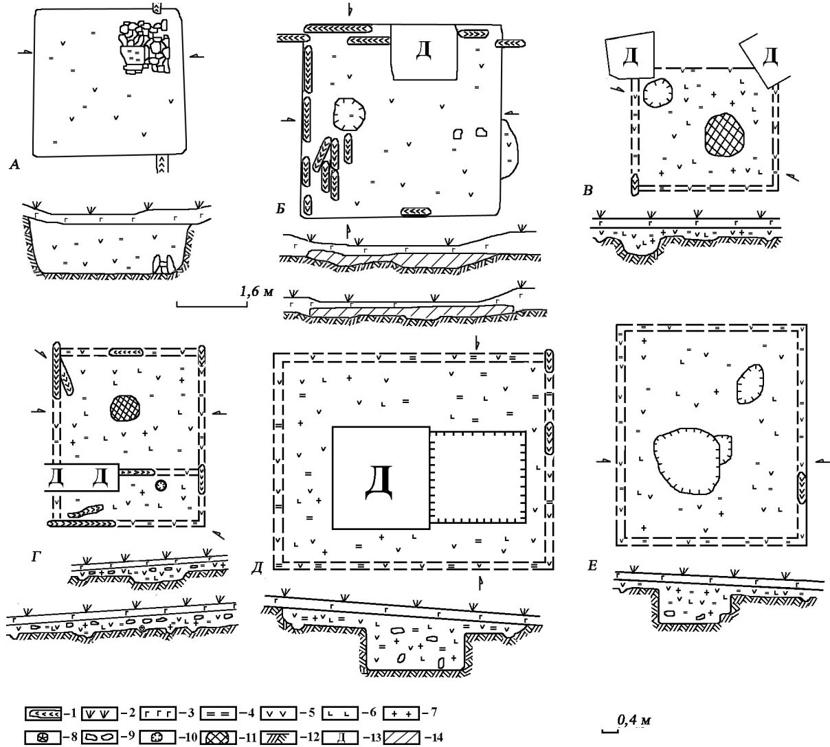
Рис. 11. Плани та профілі житлово-господарських зрубів. А–Б – Ревно (за: Тимошук, 1990, с. 60, рис. 25); В–Е – Чорнівка. 1 – обгоріле дерево; 2 – трава; 3 – гумус; 4 – обпалена земля; 5 – вугілля; 6 – кераміка; 7 – кістки; 8 – зріз дерев'яної колоди; 9 – камені; 10 – стовпові ями; 11 – черинь печі; 12 – материк; 13 – дерево; 14 – сіра земля
