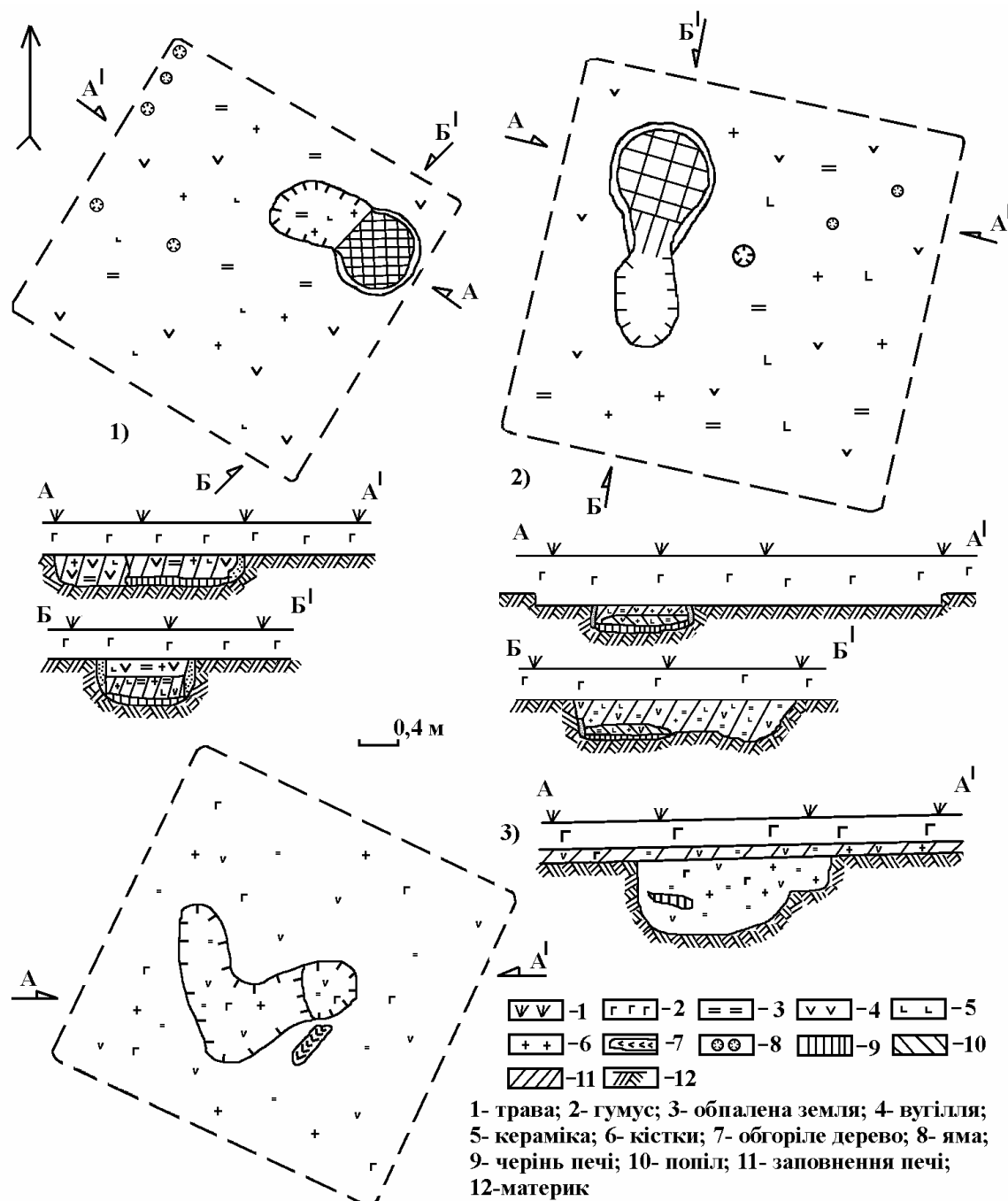
Рис. 6. Плани та профілі наземних жител з поселення Пуста Чорнівка другої половини XIII–XIV ст. 1–2 – тип 2А; 3 – тип 2Б
