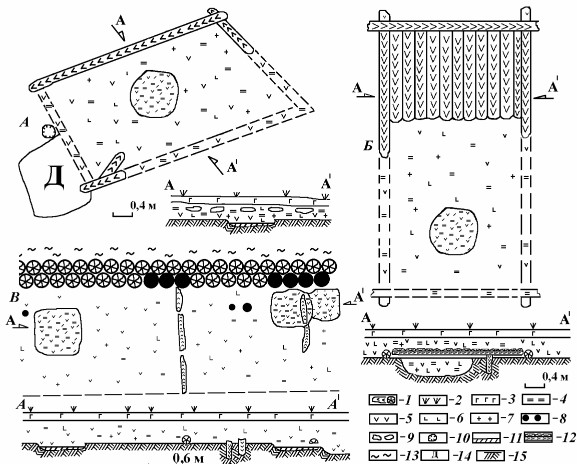
Рис. 10. Плани та профілі житлових клітей. А – Чорнівка; Б – Ленківці на Пруті (за: Тимошук, 1982, с. 75, рис. 42); В – Дарабани (Щовб) (за: Тимошук, 1971, рис. 1). 1 – обгоріле дерево; 2 – трава; 3 – гумус; 4 – обпалена земля; 5 – вугілля; 6 – кераміка; 7 – кістки; 8 – обгорілі стовпи частоколу; 9 – камені; 10 – стовпові ями; 11 – черинь печі; 12 – залишки дерев’яних нар; 13 – глина; 14 – дерево; 15 – материк
