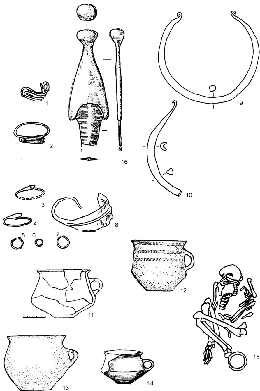
Рис. 11. Матеріали прото- і ранньоунетицького типу з Верхнього Придністров'я: 1–8 – бронзові прикраси з Передіване і Гвіздця; 9, 10 – мідні нашийні гривні з Городниці; 12, 15 – схематичний план ґрунтового поховання із с. Велика Плавуча перед Тернополем (15), керамічна посудина з цього поховання та аналогії до неї серед посуду унетицької культури (11, 13–14) Fig. 11. Materials of proto- and early-Unetice type from Upper Dnister region
